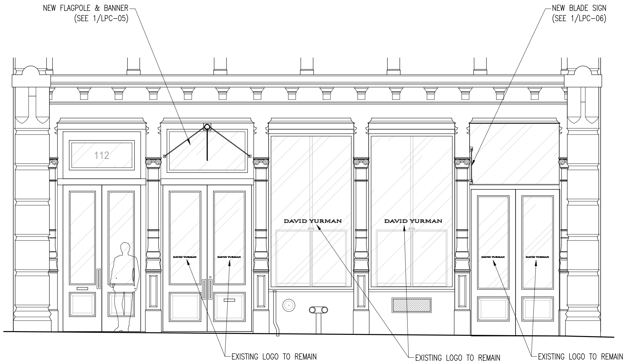
2 EXISTING STOREFRONT ELEVATION SCALE: 1/4" = 1'-0"
